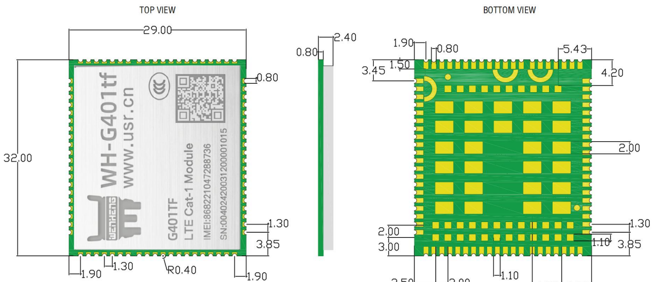
图片 17 WH-G401tf 尺寸说明
