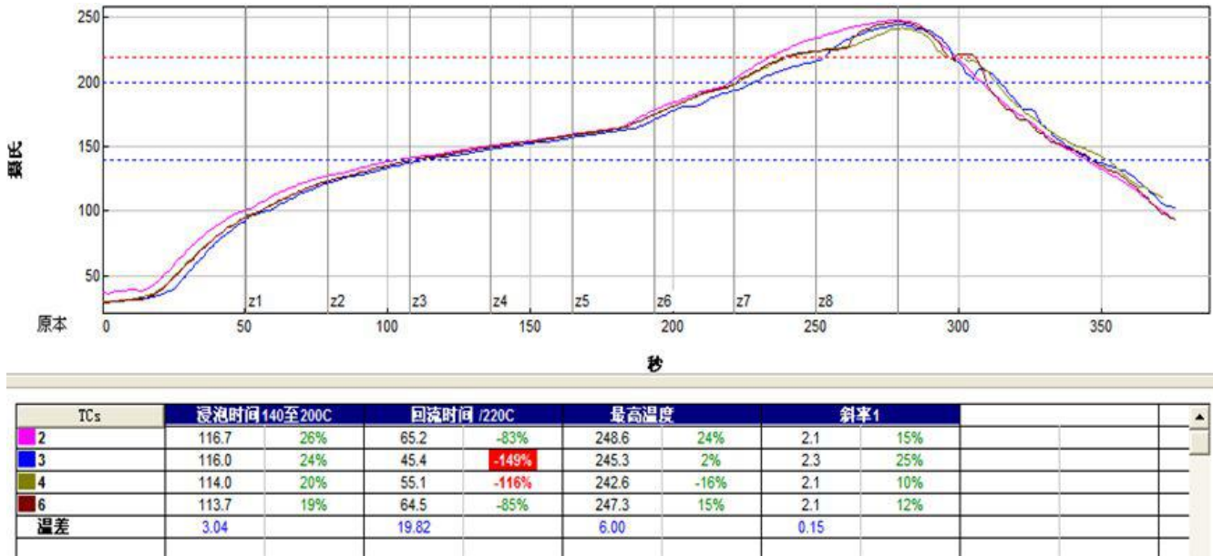
图片 16 回流焊接温度曲线图
