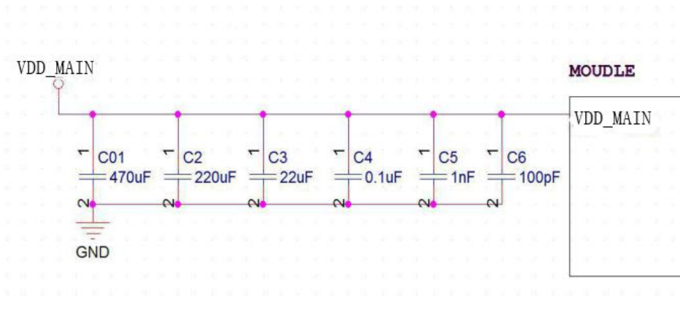
图片 4 模块电源参考电路
