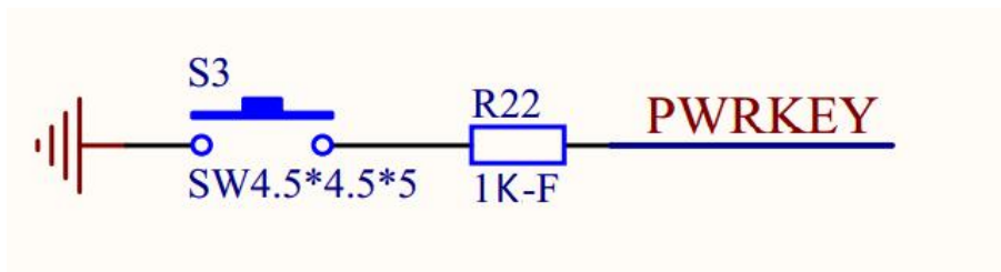
图片 14 PWRKEY 参考电路
